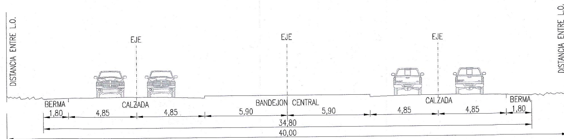
PERFIL TIPO A-A' AV. QUINTA INDUSTRIAL Esc. S/E
