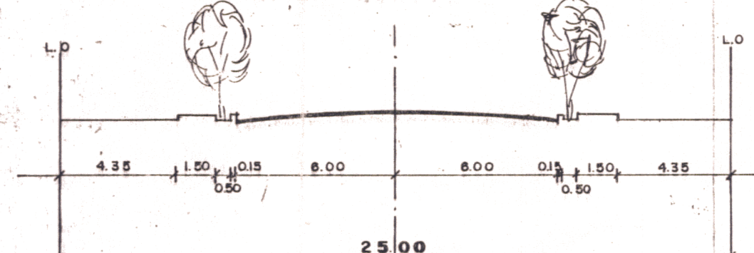
PERFIL C'-C
